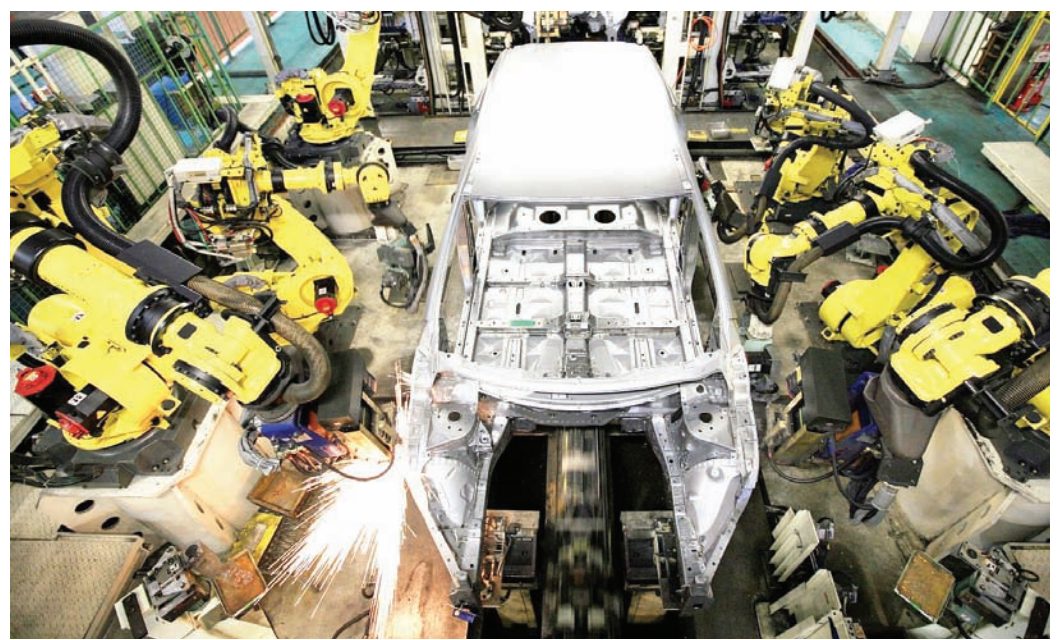
Robots en plena labor en una de las 14 plantas de producción de vehículos Toyota en Estados Unidos, que continuamente son modernizadas para que sus unidades sigan como líderes de la industria automotriz. FOTO: TOYOTA
